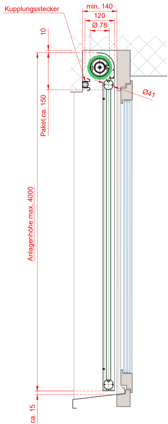
Mögliches Anschlussdetail
