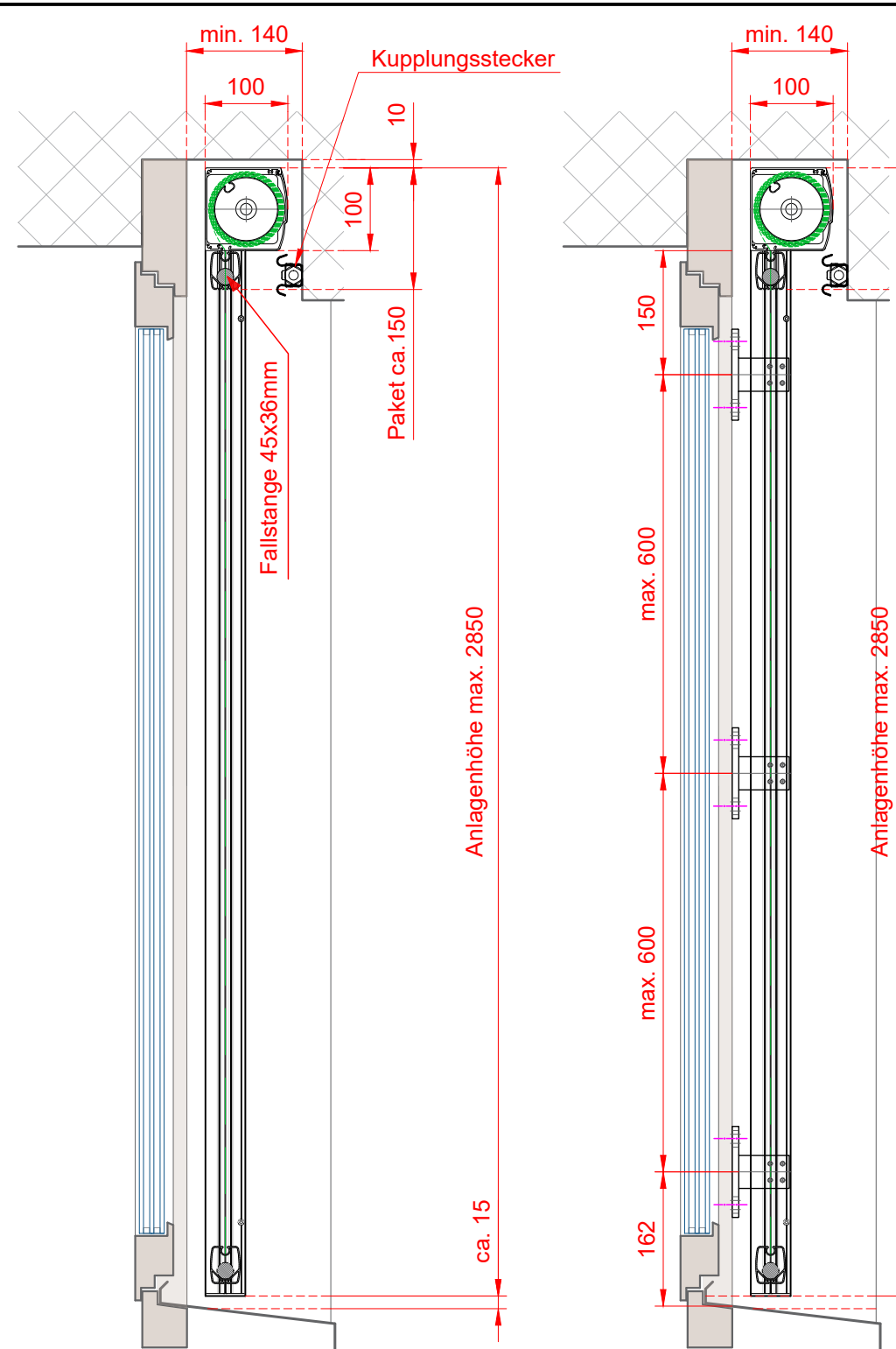
Montage T-Stütze
