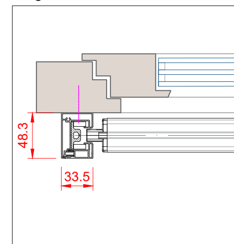
Mögliches Anschlussdetail
