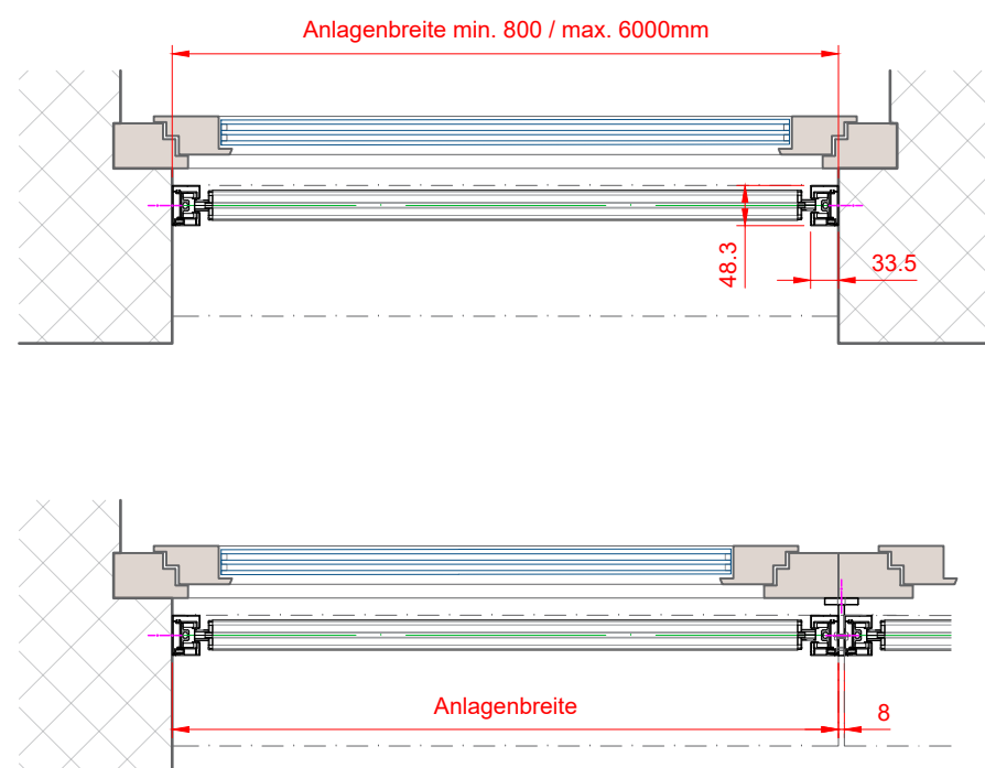
Mögliches Anschlussdetail
