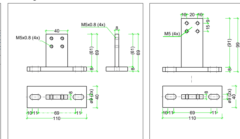
Montage T-Stütze
