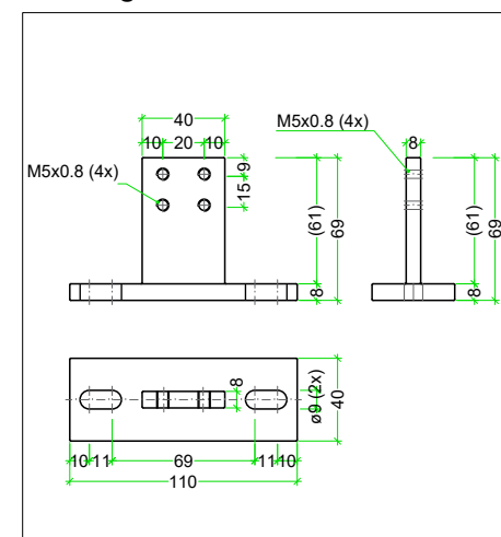
Montage T-Stütze
