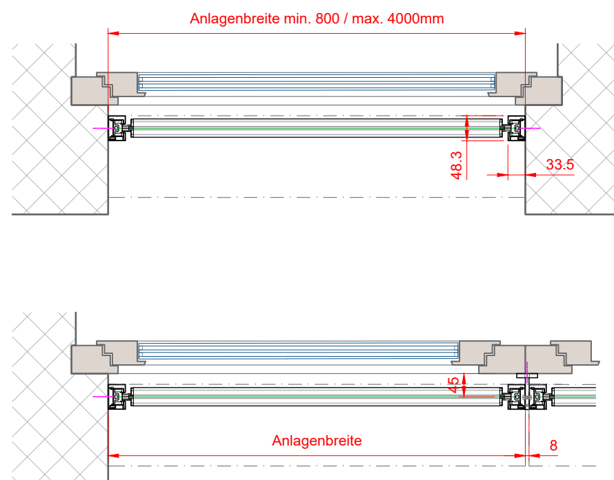
Mögliches Anschlussdetail
