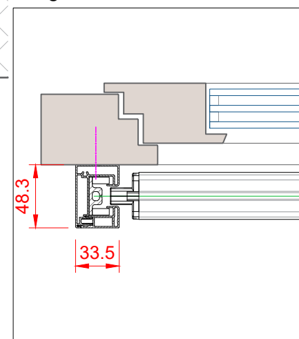
Mögliches Anschlussdetail
