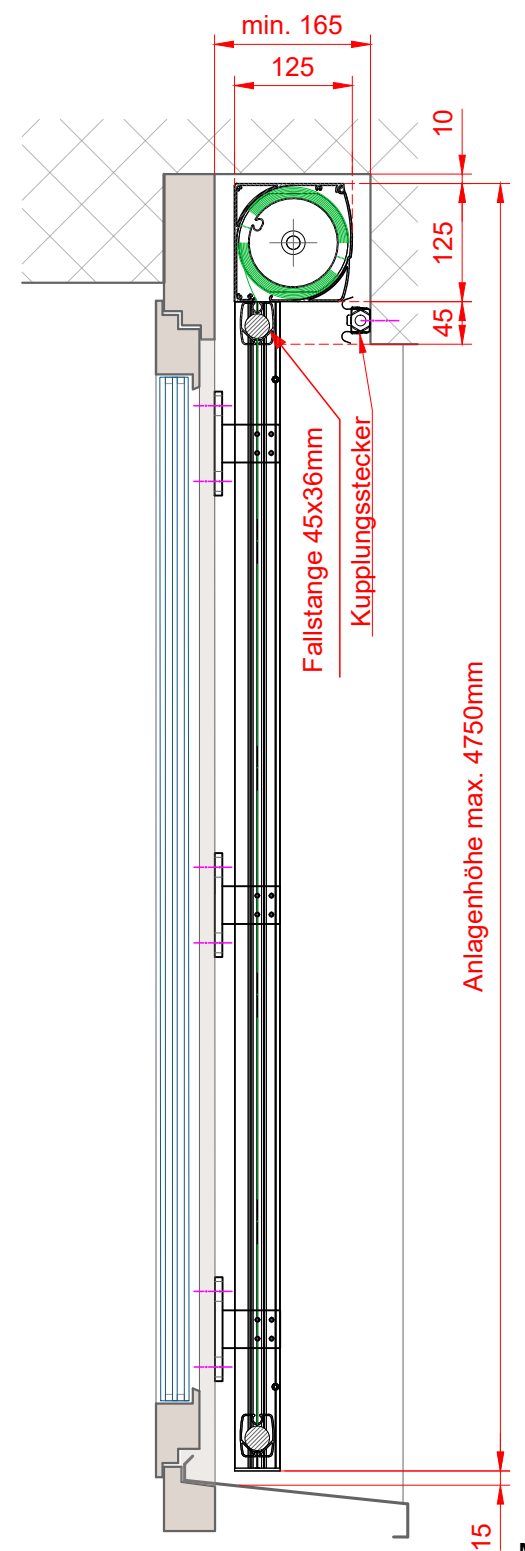
Mögliches Anschlussdetail
