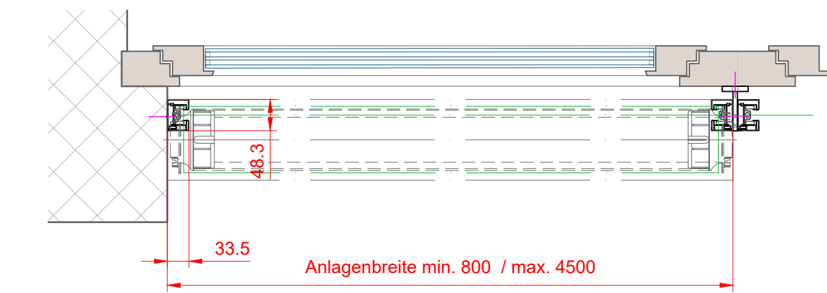
Mögliches Anschlussdetail
