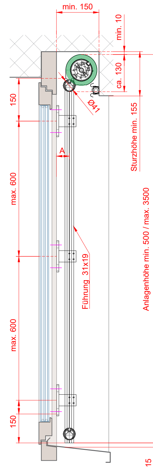
Montage T-Stütze: A = 45 / 60 / 75 / 90mm (Standard)
