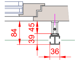
Mögliches Anschlussdetail
