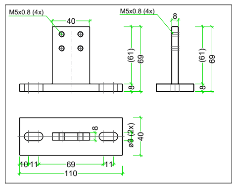
Montage T-Stütze: A = 45 / 60 / 75 / 90mm (Standard)
