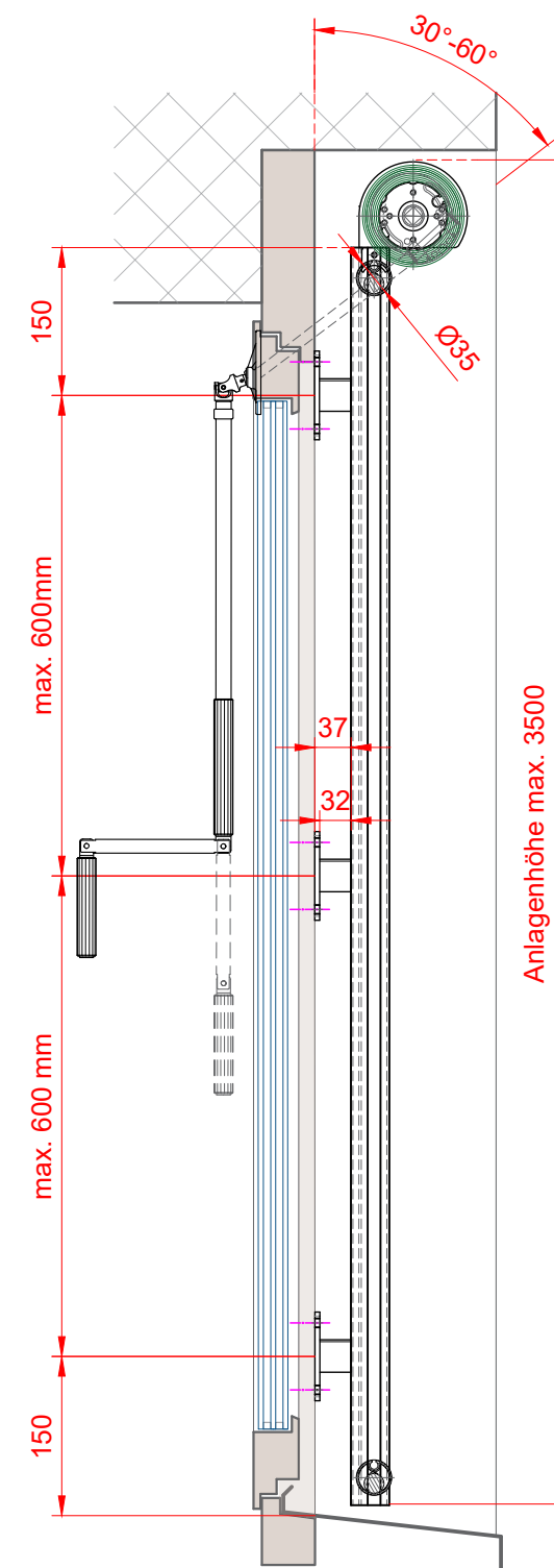
Mögliches Anschlussdetail
