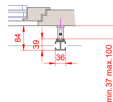
Mögliches Anschlussdetail
