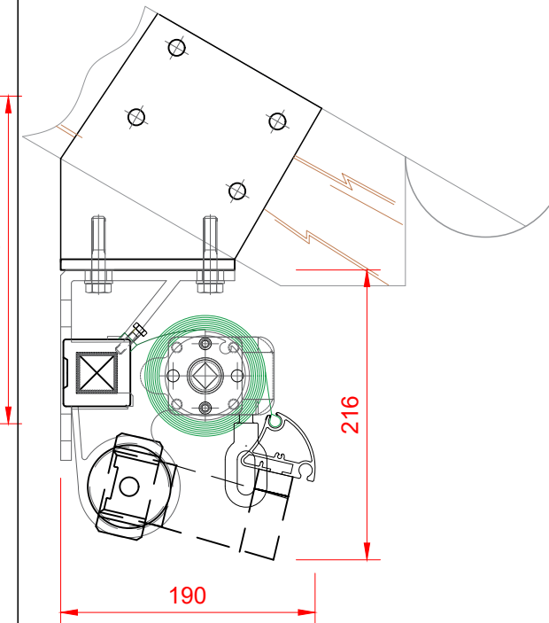
Montage auf Dachsparren
